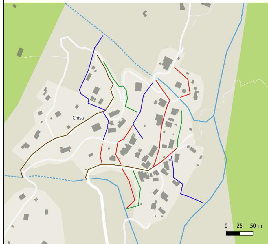
Canaux d'irrigation par voie gravitaire
